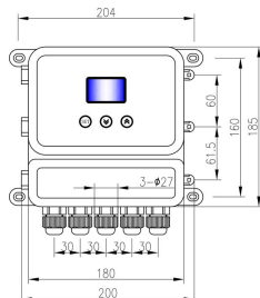
图 4 明渠流量计结构图
