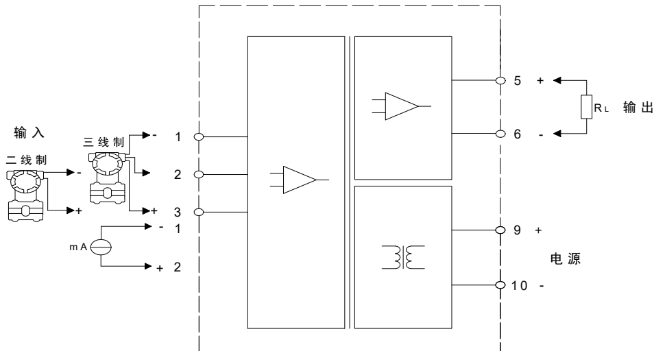
图 2 单入单出电流输入接线图
